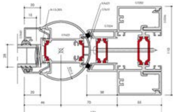
Thermal Profile
